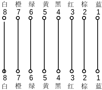
芯线接法(1:1)
